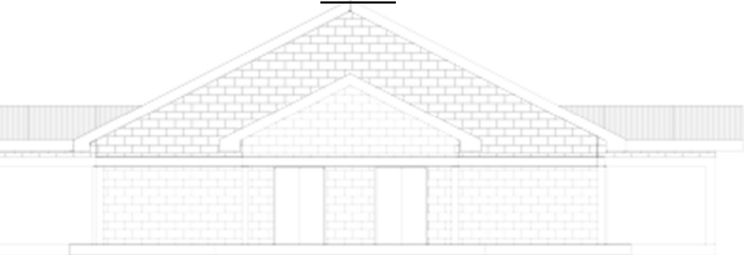
Elevation 02
